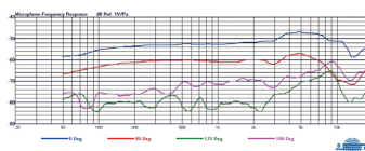
MU-90 頻響圖
